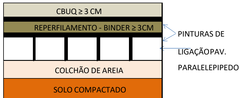
CORTE GENÉRICO 02
